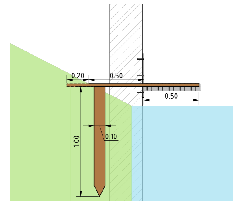
Voorbeeld Schaal 1:20
