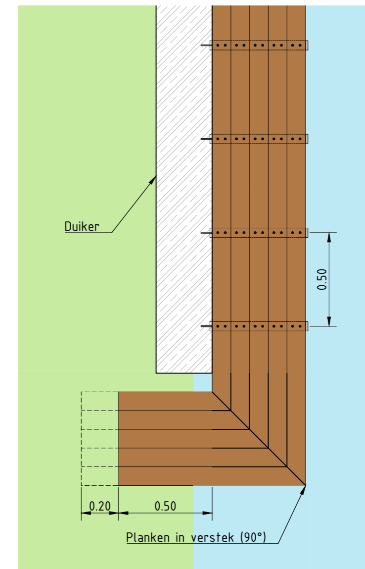
Bovenaanzicht Schaal 1:20
